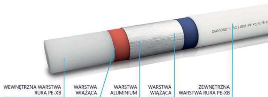
Fot. 1. Rura PEX – widok warstw
